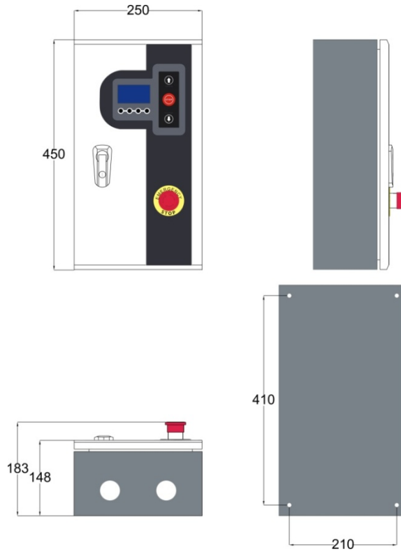
1.5KW Controller
