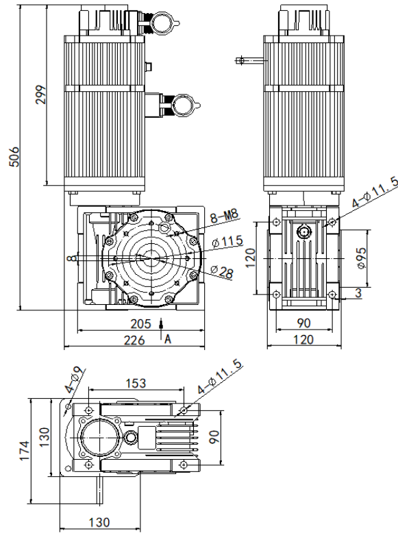
2.2KW Motor
