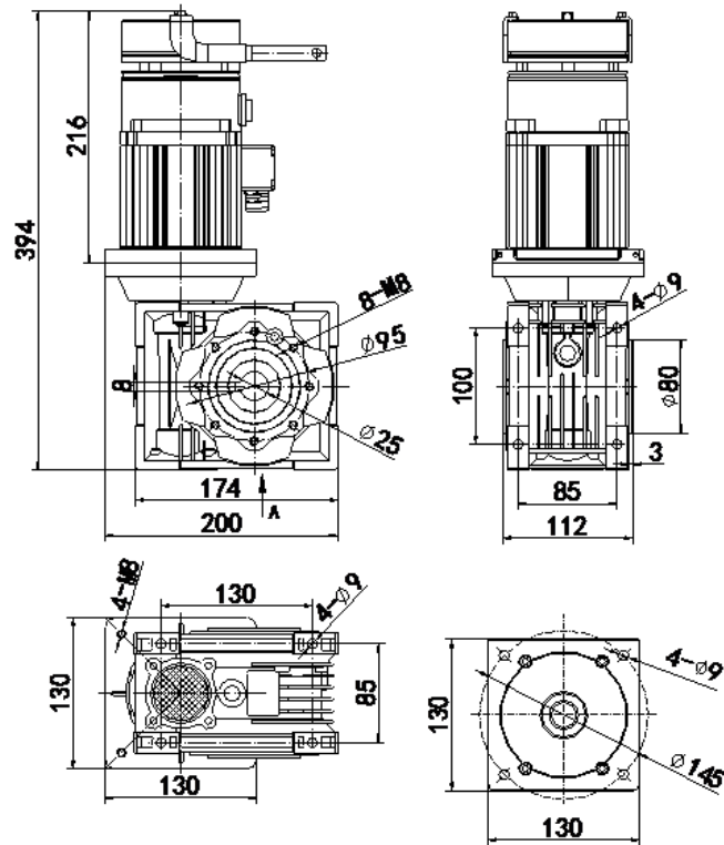
1.5KW Motor
